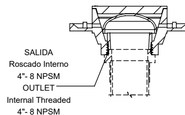
SECCIÓN A-A A-A SECTION
