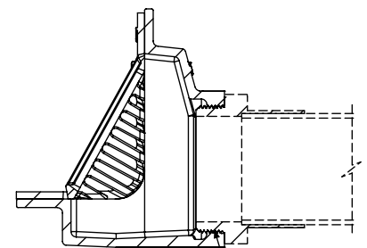
SECCIÓN A-A A-A SECTION
